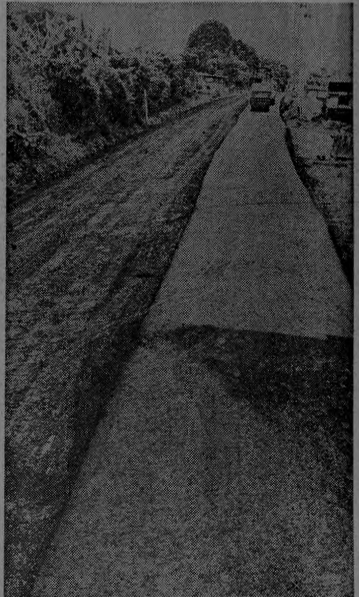
Una aplanadora tipo tandem, especial para este trabajo, se ve al fondo en labor de aplanchado y compactación de la carpeta asfáltica, que minutos antes hubiera colocado la terminadora de asfalto. Se aprecia en el grabado un carril de la Calle de la Guacamaya terminado, y el otro listo para recibir la mezcla asfáltica. — (foto Córdoba)
